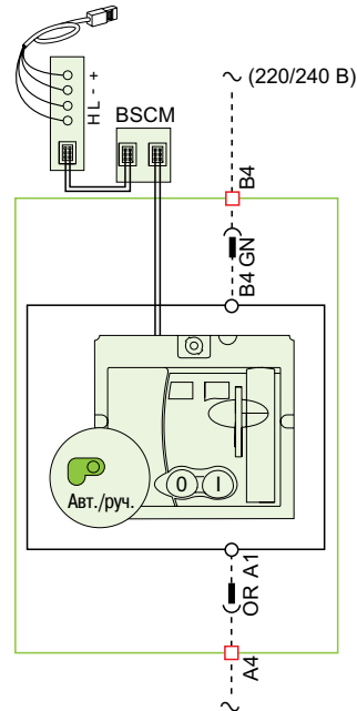
Коммутационный мотор-редуктор (MTc) (1)
