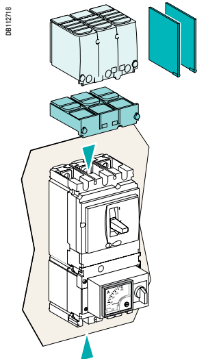
Выключатель с блоком амперметра
