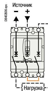
Последовательно подключение возможно на вводе или отходящих линиях (осуществляется пользователем)
