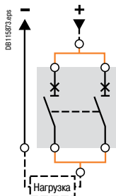
Выбор 3 : 2-полюсный Compact NSX100N DC с параллельным подключением полюсов
