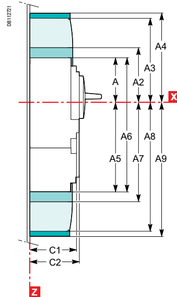
NSX100 - 630
