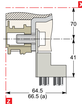
NSX100 - 250
