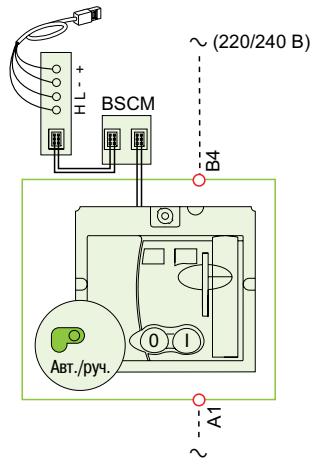
Коммутиционный мотор-редуктор (МТс) (1)
