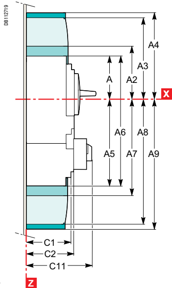
NSX100 - 250
