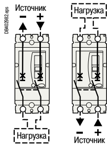
Верхнее или нижнее подсоединение ввода и отходящих линий
