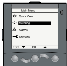
Дисплей щитового индикатора FDM121: перемещение по меню
