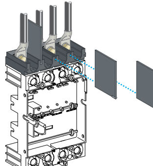
Переходник для цоколя 4-полюсного аппарата 400/630 A. Присоединение расширителей полюсов с разделителями полюсов
