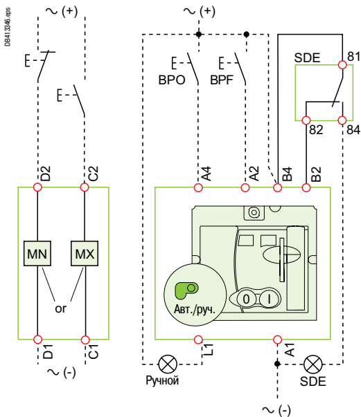
Мотор-редуктор (МТ)
