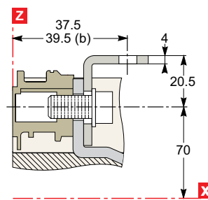
NSX100 - 250
