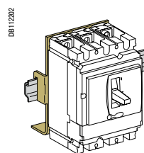
Крепление на DIN-рейке при помощи переходника
