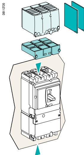
Выключатель с блоком трансформатора тока
